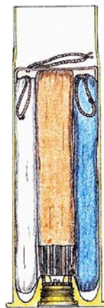
État final à partir de 1937 environ. Charges partielles de poudre en bandes dans de longs sachets.
