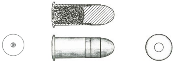
La première cartouche en métal à allumage annulaire centrale Ordonnance 1878.
