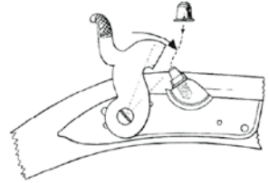
Amorce à percussion avec capsule.
